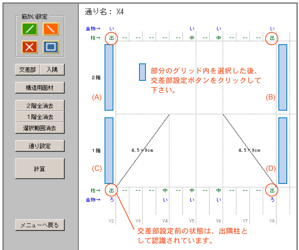
図3.3.3 軸組の選択範囲
