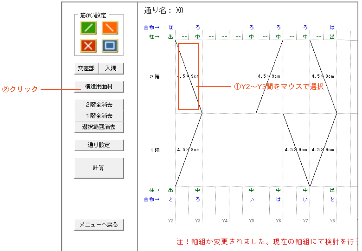
図3.3.6 面材の設定
